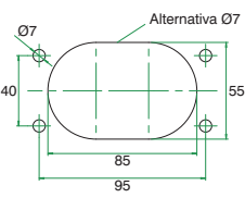
Schema di foratura
