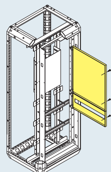
PLACCHE FRONTALI CIECHE E FORATE
