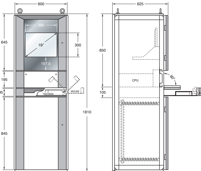
DRC-LAN-B.35 con antina ribaltabile e cassetto estraibile
