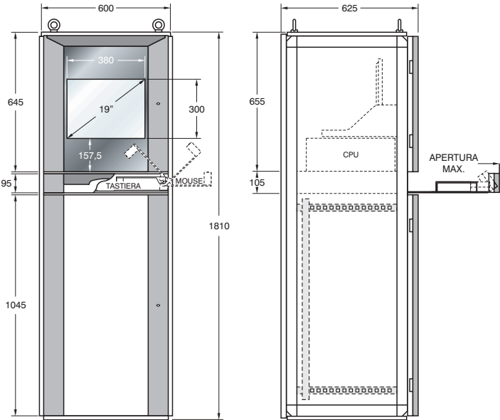
DRC-LAN-A.35 con cassetto centrale estraibile
