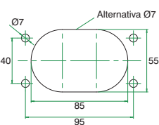
Schema di foratura
