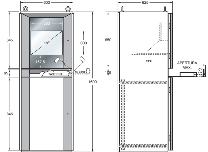
DRC-LAN-1/A con cassetto centrale estraibile
