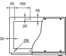
FLANGIA INGRESSO CAVI
