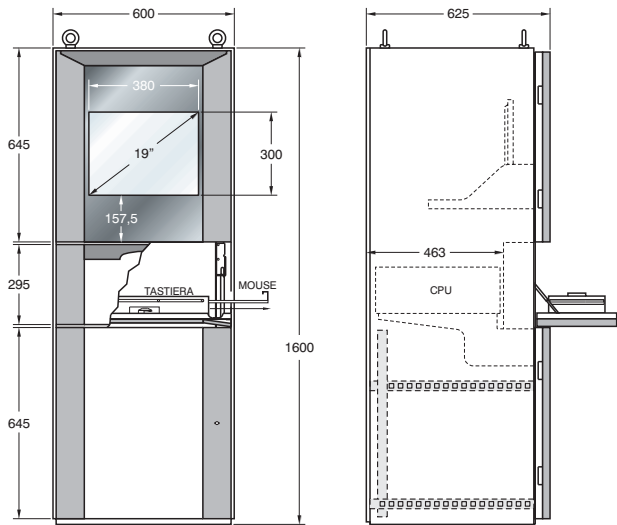
DRC-LAN-1 con antenna ribaltabile
