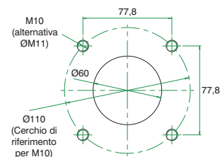
Schema di foratura
