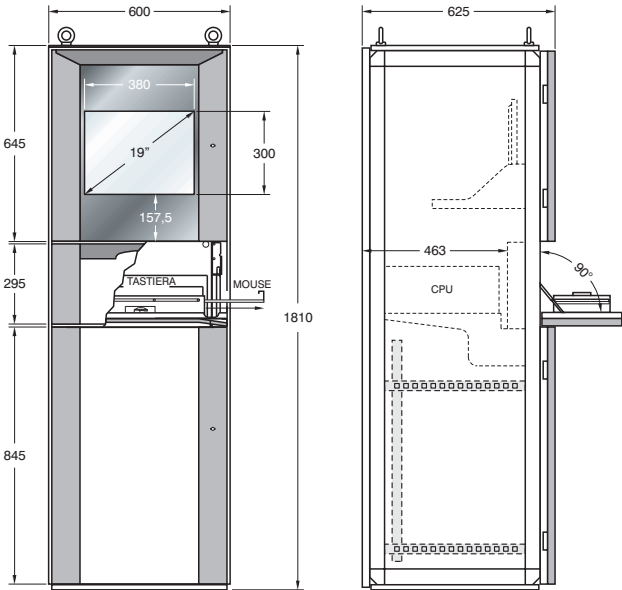
DRC-LAN.35 con antina ribaltabile
